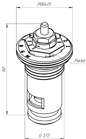
Рисунок 1 – Габаритные размеры
